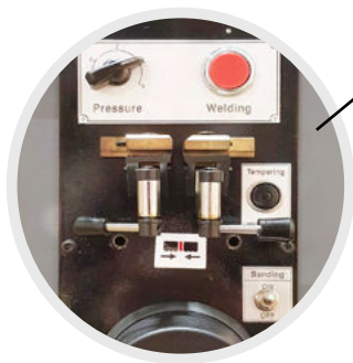
Knip-, las- en slijpinrichting t.b.v. lintzaagblad
